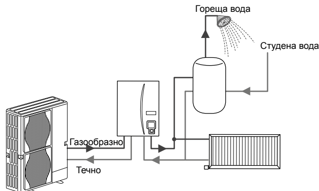
Изображение на термopомпената система с Hydrobox
