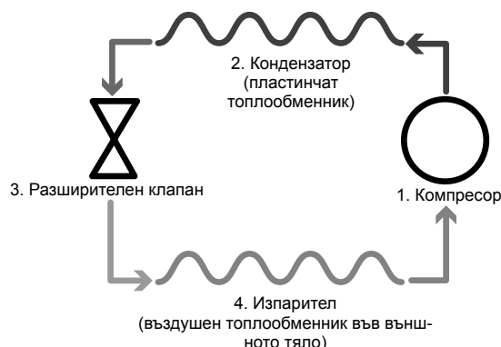
Изображение на термopомпената система с Hydrobox
